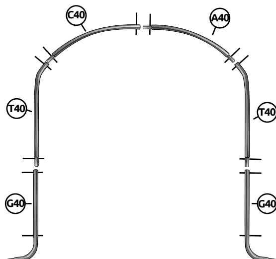
Vue de l'arceau
